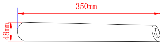
Leg (2) Qty:4
