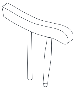
RIGHT ARM (B2) Qty: 1 355 x 319 x 43 mm
